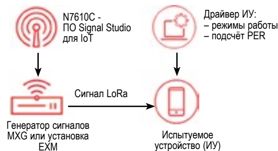
Рисунок 3. Схема стенда для испытаний приёмного тракта.
