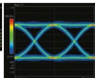
Глазковая диаграмма
